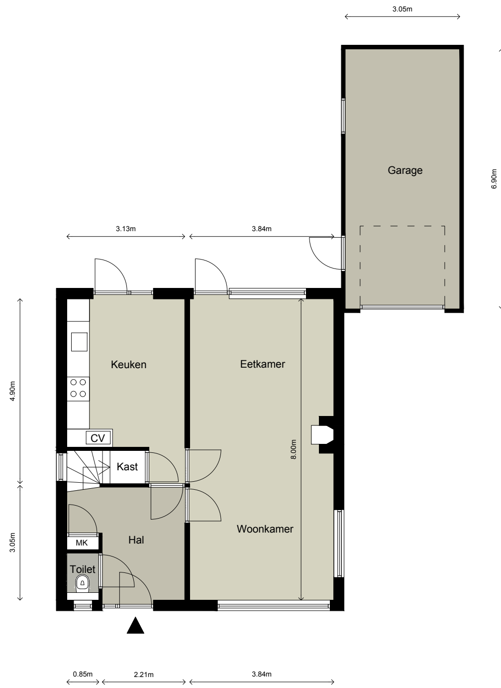
Begane grond
