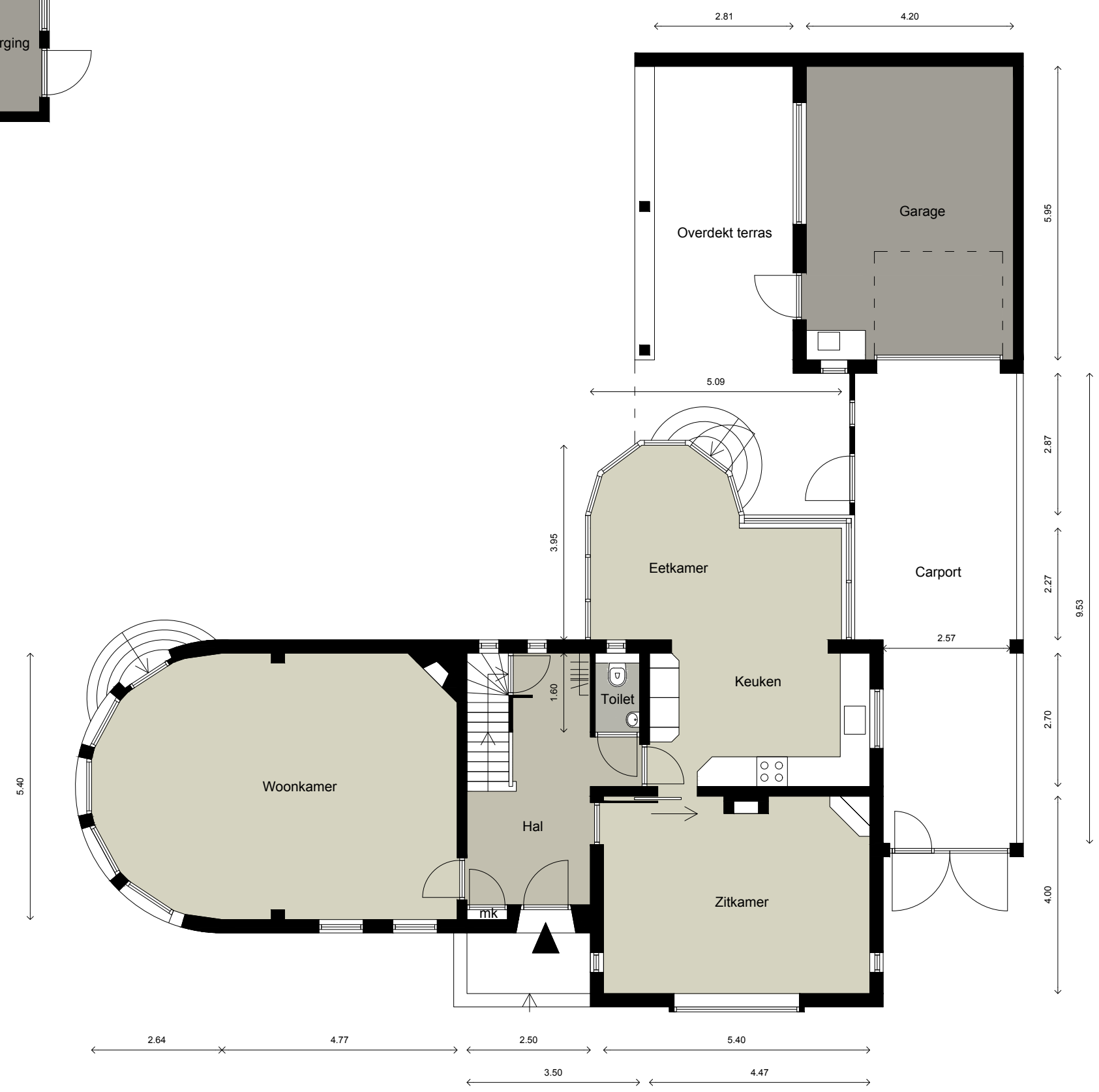
Begane grond
