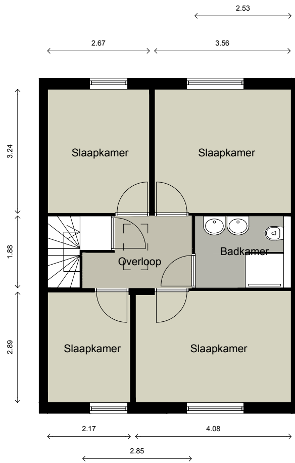
Eerste verdieping
