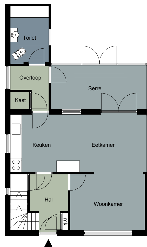
Begane grond
