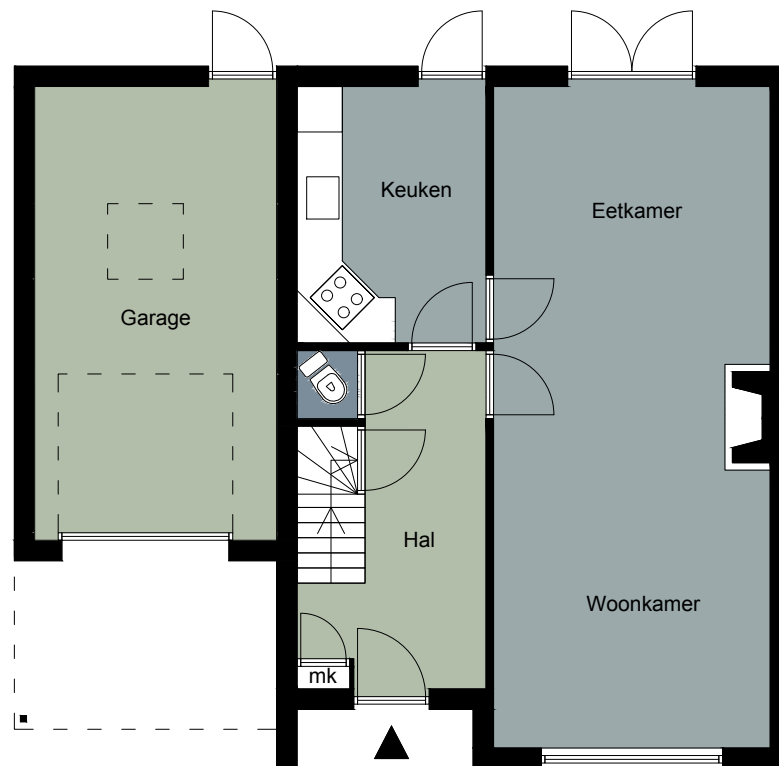
Begane grond
