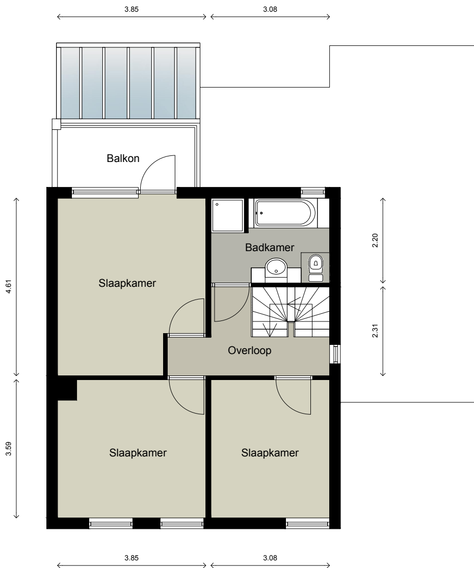
Eerste verdieping
